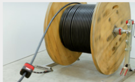
RM35 mit RUNPOLIFTER L1600 und 3 x 35 mm 2 Kabel RM35 with RUNPOLIFTER L1600 and 3 x 35 mm 2 cable
